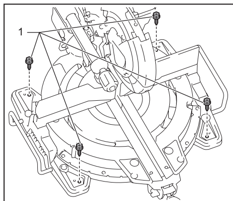
► 1. Bolts
