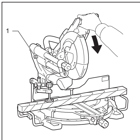
► 1. Stopper pin
